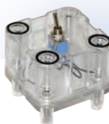
Commutateur Interrupteur inverseur à levier U max : 24 V I max : 3 A Réf. P/DQ047 Prix TTC : 21,10 €
