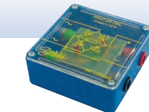
Pont de DEL Umax = 12 V Réf. P/CSS0042 Prix TTC : 21,50 €
