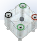
Pont de diodes U max : 100 V I max : 1,5 A Réf. P/DQ040 Prix TTC : 15,80 €
