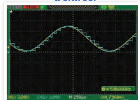
Fréquence d'échantillonnage moyenne par rapport au signal d'entrée
